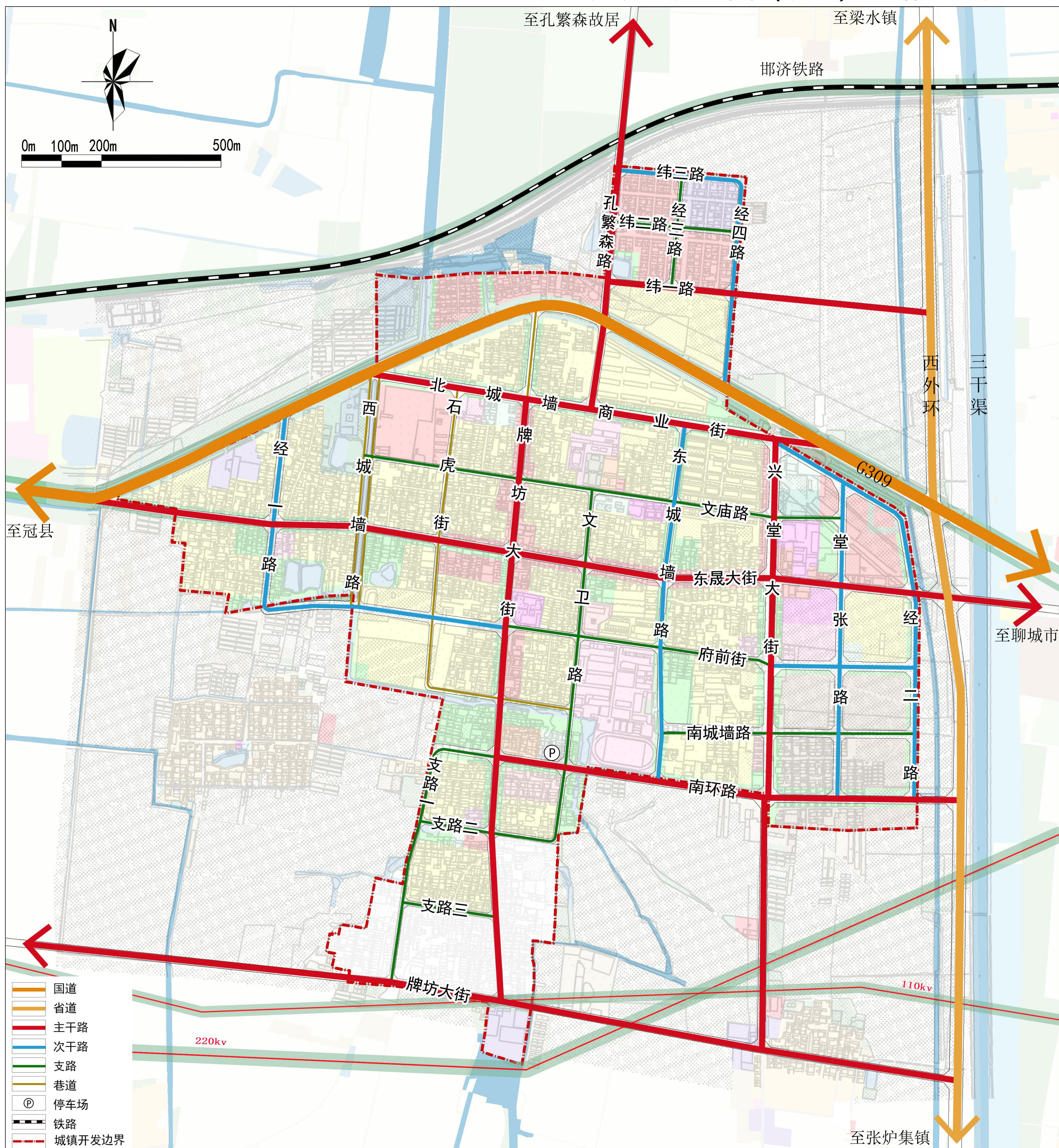
城镇开发边界范围（镇区）道路交通规划图
