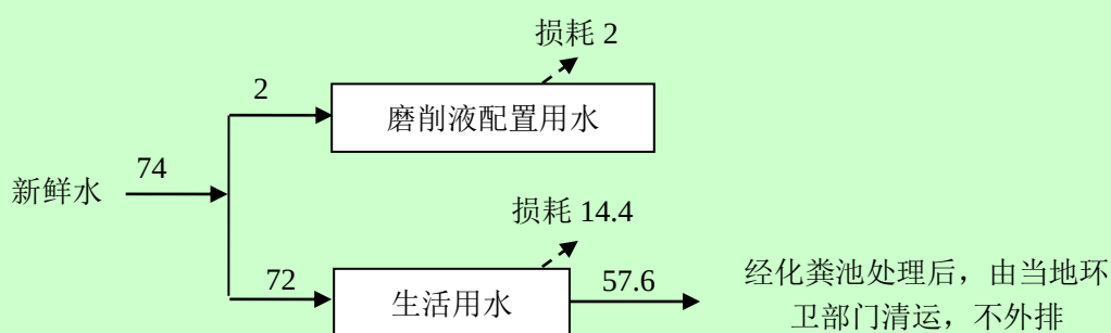
图 1 项目水平衡图 (m 3 /a)
