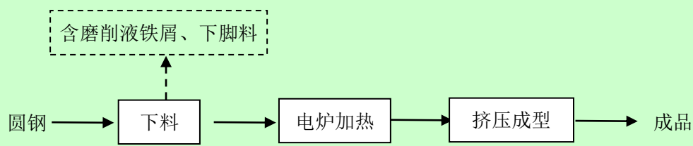
图 2 项目生产工艺流程及产污环节图
